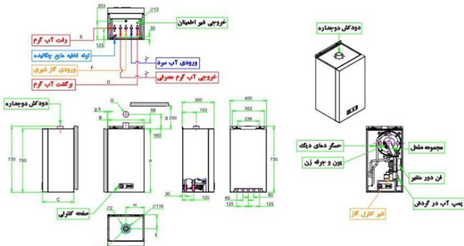
اندازه‌های محل نصب بر اساس سری ساخت
